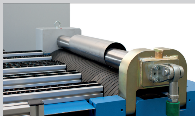
Klapplager / Bearing cap
